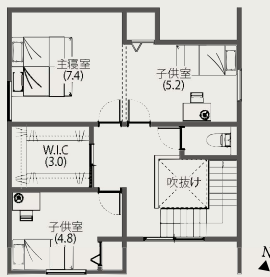
2F
